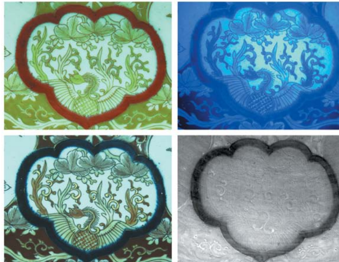
IMAGISTICĂ MULTISPECTRALĂ
